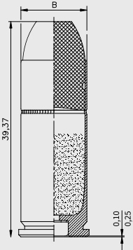
Desenho ilustrativo da altura e profundidade do espoletamento.
