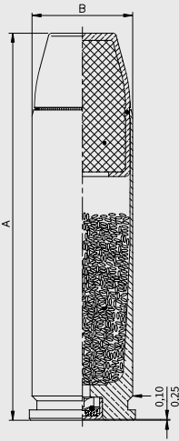
Desenho ilustrativo da altura e profundidade do espoletamento.
